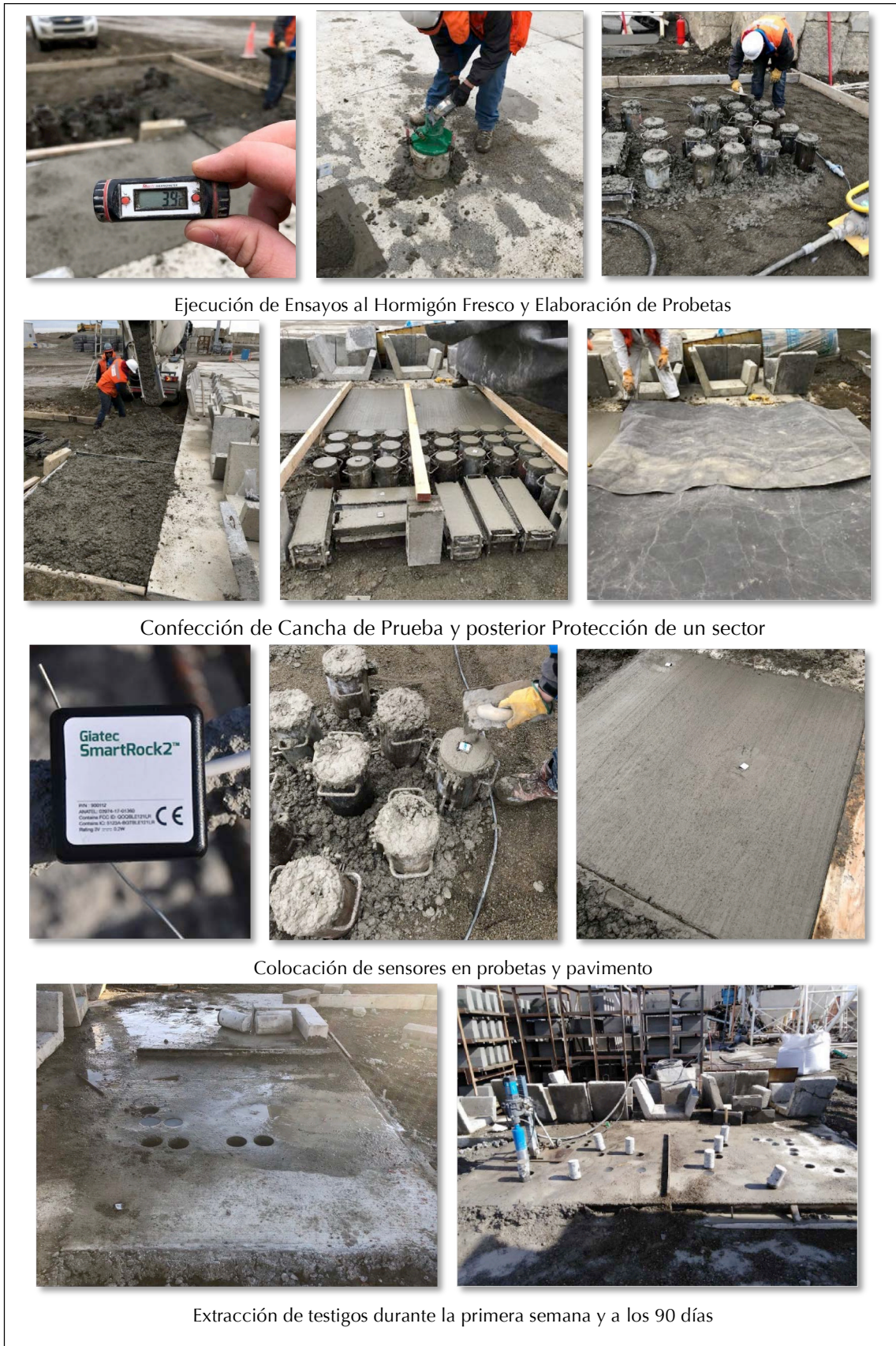
Figura 7. Proceso completo de la actividad de medición de Madurez y Estimación de Resistencia
