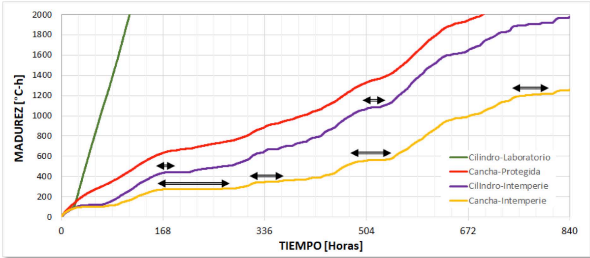
Figura 10. Desarrollo de la Madurez en las Probetas y Cancha de Prueba para T_o=0^{\circ}\text{C}
