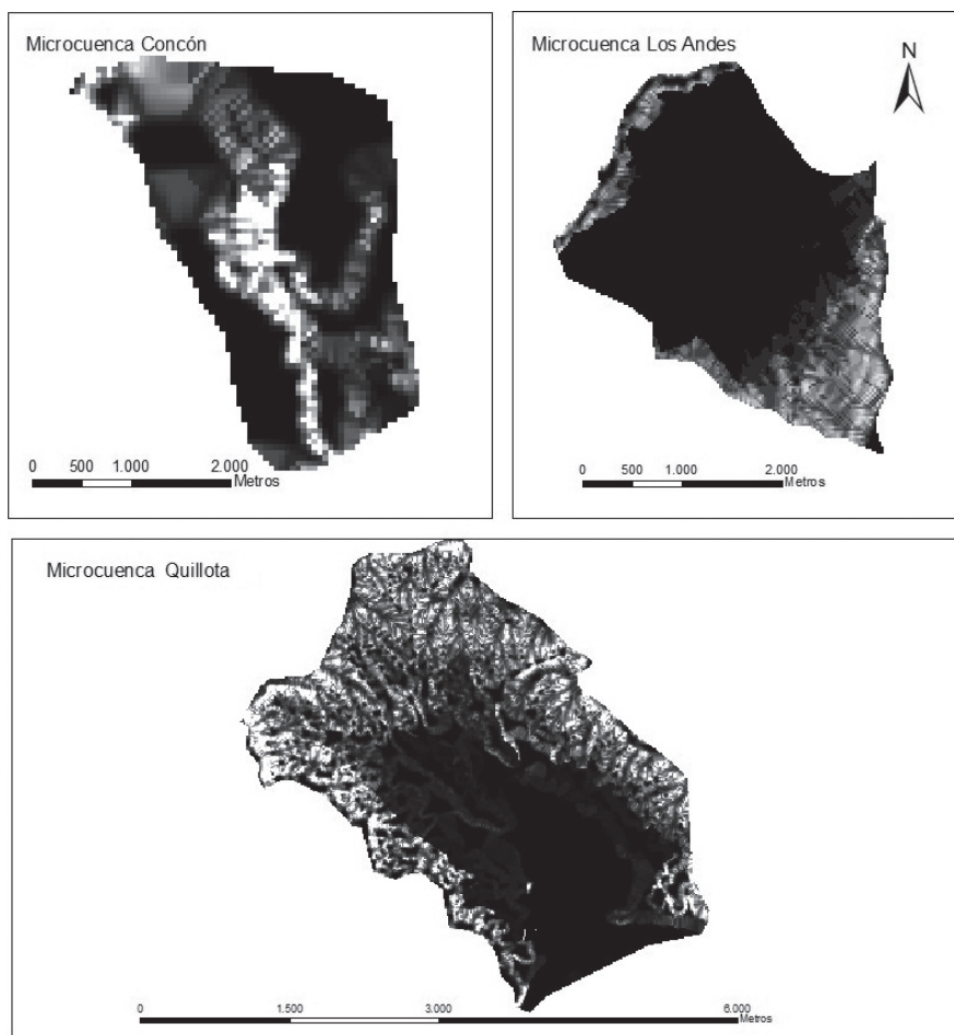
Figura N° 4 Pérdida de suelo según USLE, aplicada a las comunas de Los Andes, Quillota y Concón
