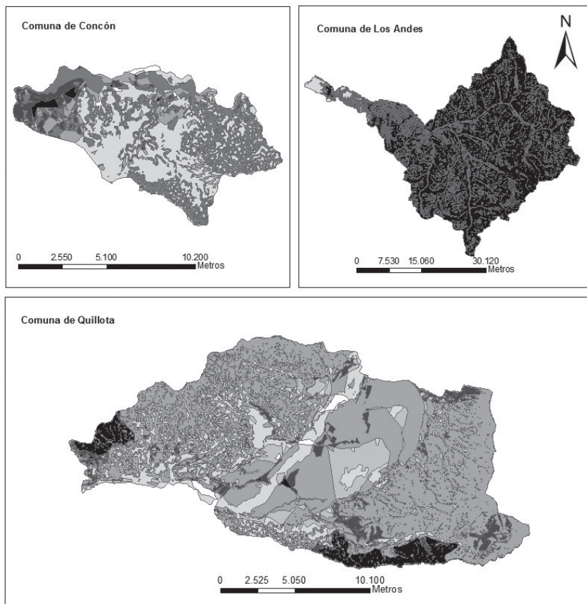
Figura N° 3 Unidades de Respuesta a la Erosión (ERU) en las comunas de Los Andes, Quillota y Concón
